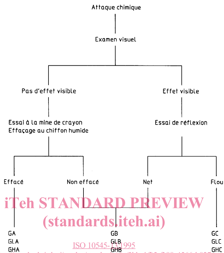
Figure 1 — Schéma de classification pour la résistance chimique des carreaux émaillés
