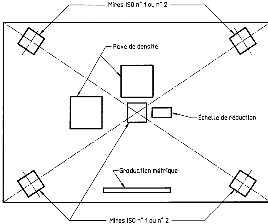
Figure 1 — Cible de contrôle (standards.itech.ai)
