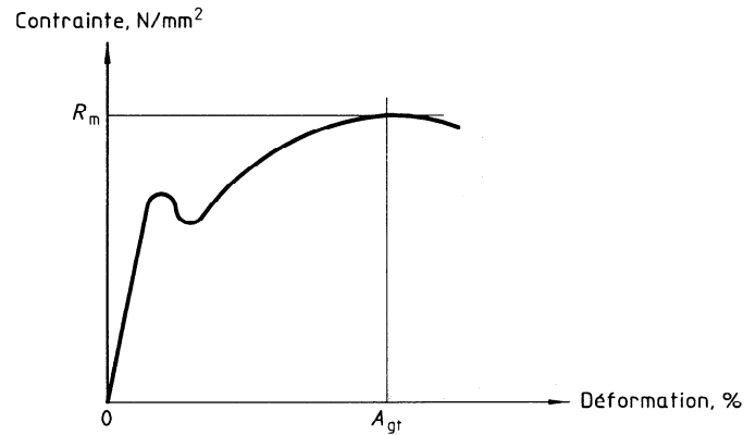
Figure 1 — Exemple de courbe contrainte/déformation
