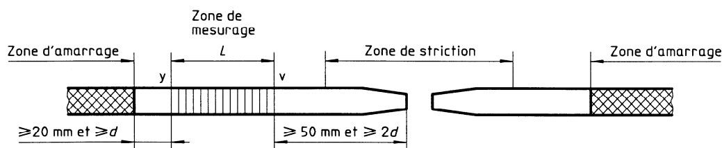
Figure 2 — Mesurage après rupture
