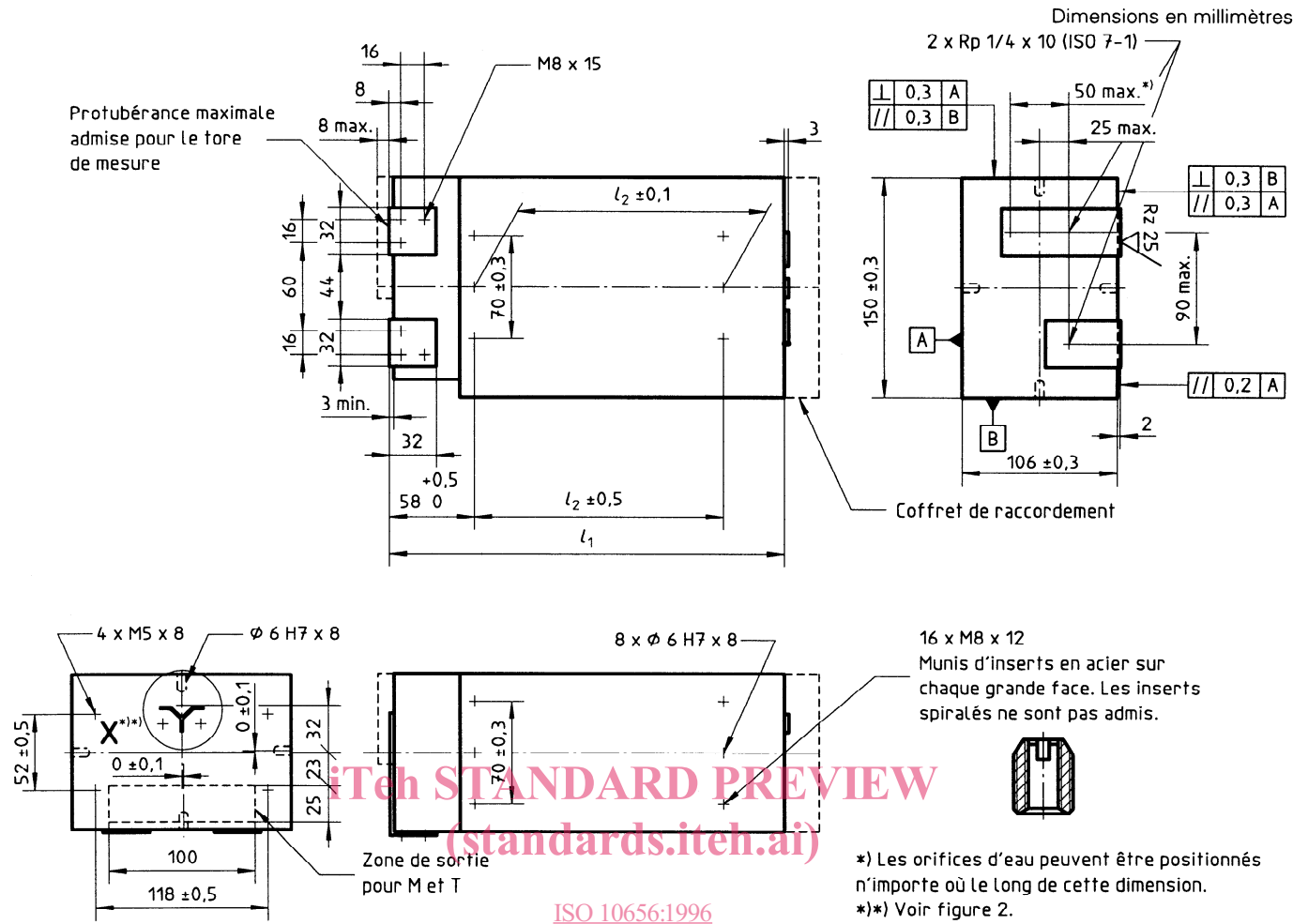
ISO 10656:1996 http://standards.iteh.ai/catalog/standards/iso-10656-1996/b28a226fa7fe/iso-10656-1996 Figure 1 — Dimensions des transformateurs de type H
