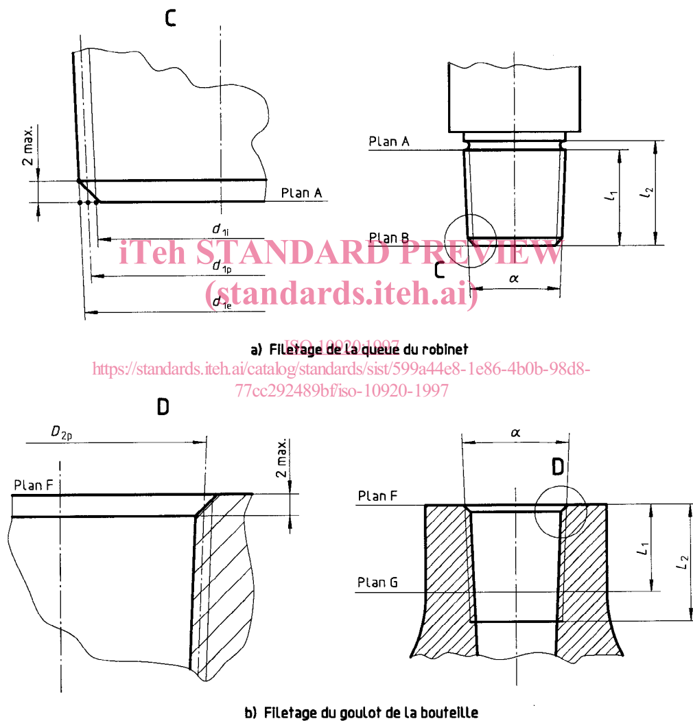
Figure 1 — Plans de référence et diamètres des filetages
