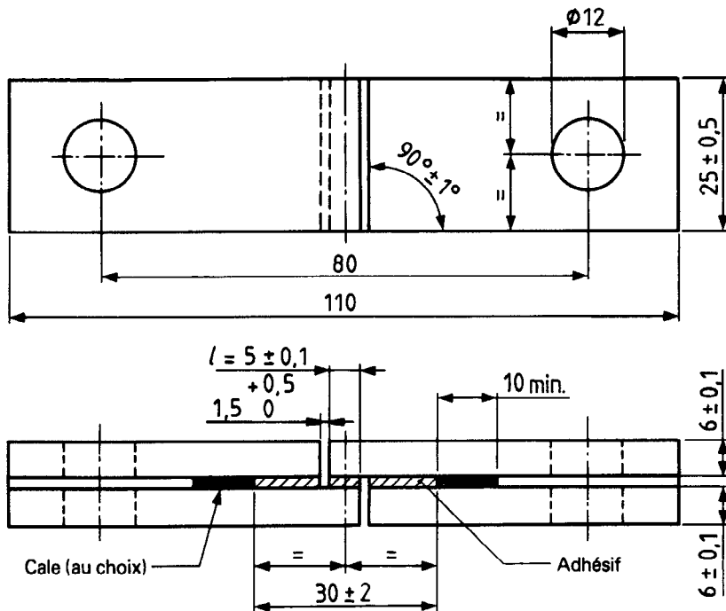
Figure 4 — Éprouvette
