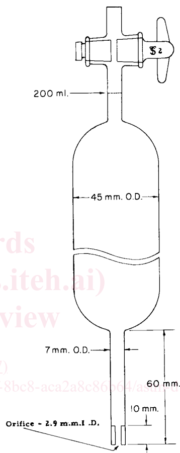
FIG. 1 Foam Pipet
