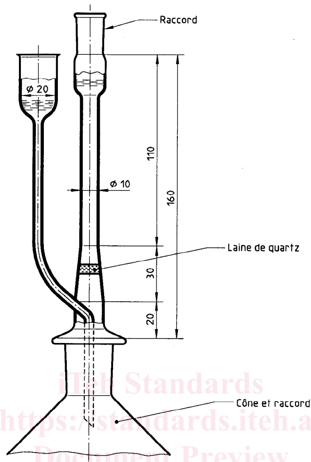
Figure 1 — Microséparateur
