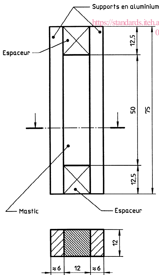
Figure 1 — Montage des éprouvettes d'essai
