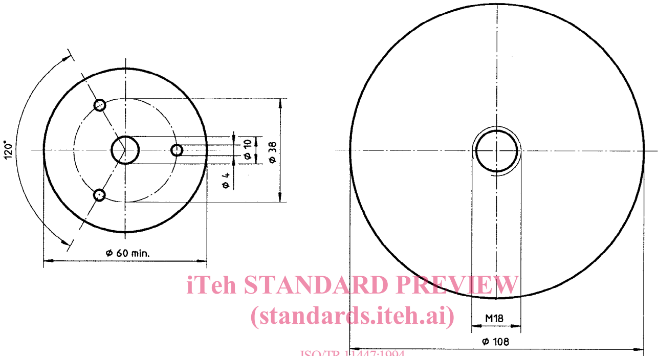
ISO/TR 11447:1994 https://standards.iteh.ai/catalog/standards/sist/9804ee73-0023-40ba-a9de-f8b96ce3693f/iso-tr-11447-1994 a) Fixation sur base de type A b) Fixation sur base de type B
