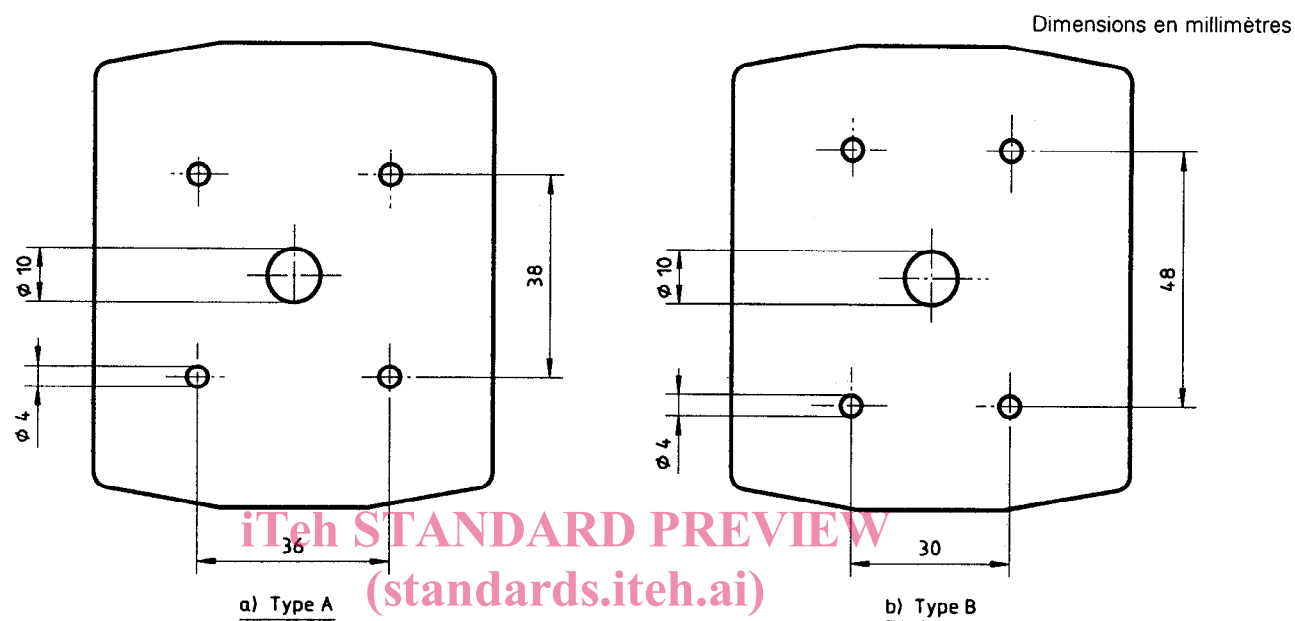
Figure 2 — Navires de moins de 12 m de longueur — Feux autres que les feux de tête de mât ISO/TR 11447:1994 https://standards.iteh.ai/catalog/standards/sist/9804ce73-0023-40ba-a9de-f8b96ce3693f/iso-tr-11447-1994
