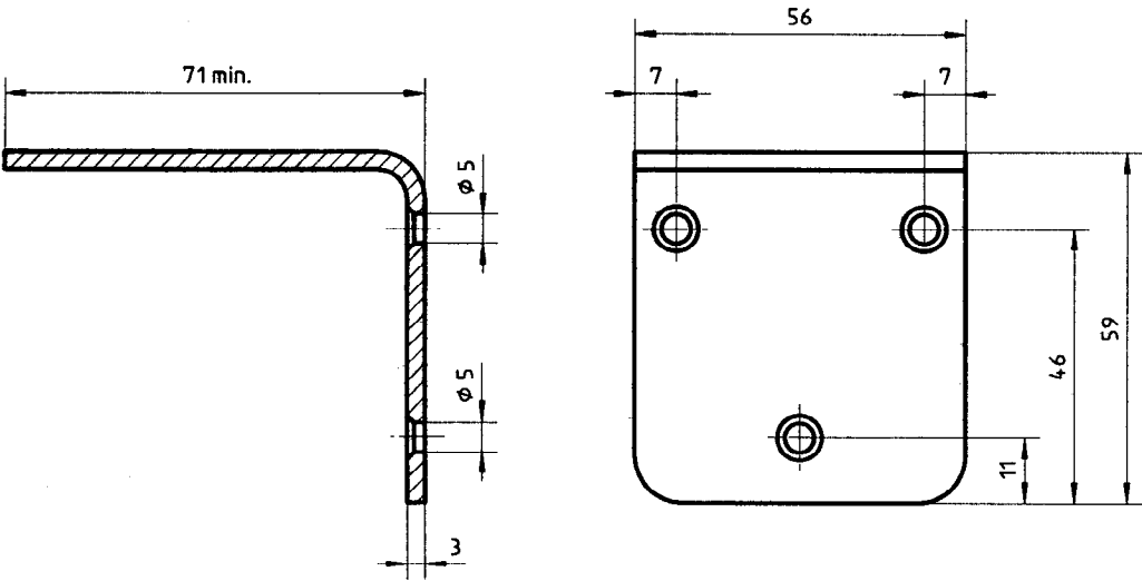
c) Fixation en applique (type C)
