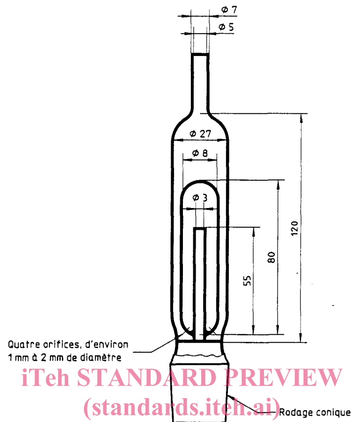
Figure 2 — Exemple de chambre d'absorption https://standards.iteh.ai/catalog/standards/sist/a35add3c-2392-43eb-9925-e80ebe7f68b6/iso-11466-1995
