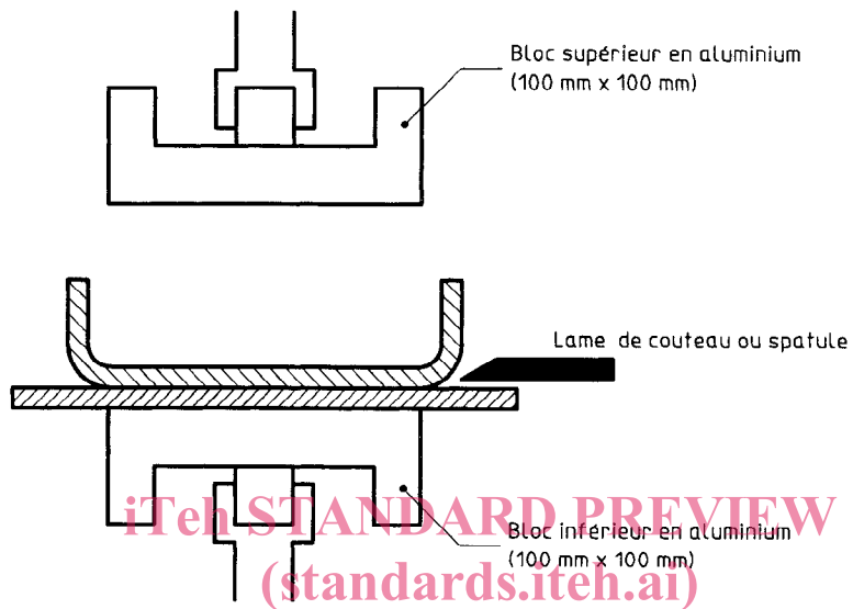
Figure 4 — Fixation des éprouvettes bloquées sur les blocs en aluminium dans la méthode quantitative
