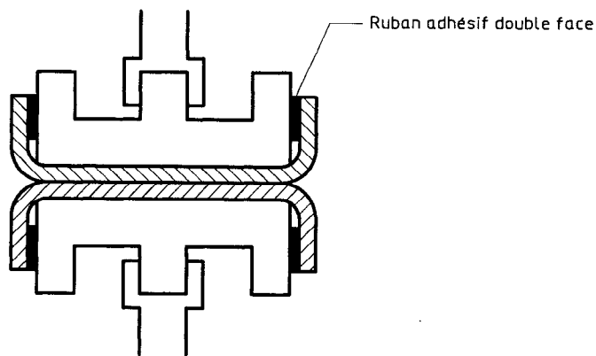
Figure 5 — Éprouvette en place pour l'essai dans la méthode quantitative (méthode B)
