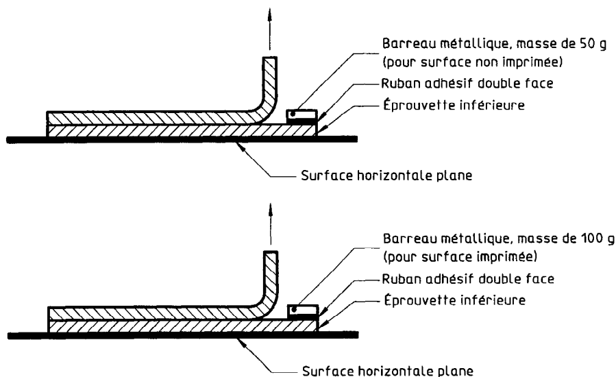
Figure 2 — Séparation des éprouvettes dans la méthode qualitative (méthode A)
