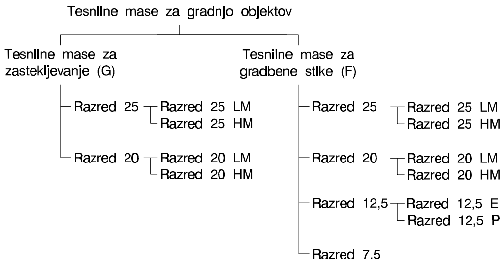
Slika 1: Diagram razdelitve tesnilnih mas za gradnjo objektov
