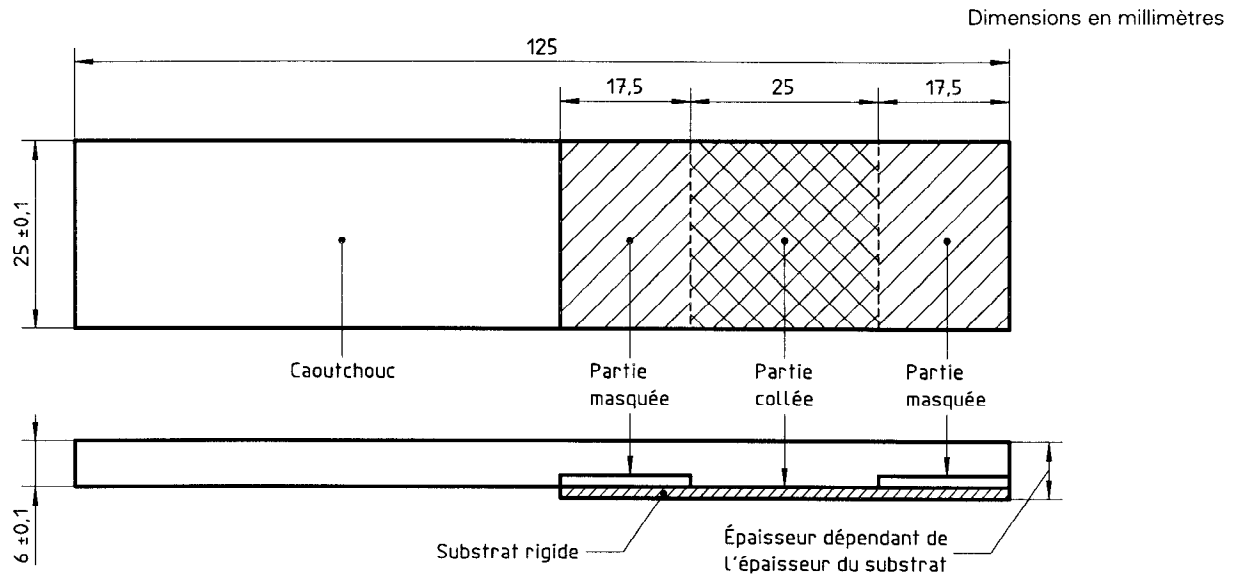
Figure 2 — Éprouvette normalisée
