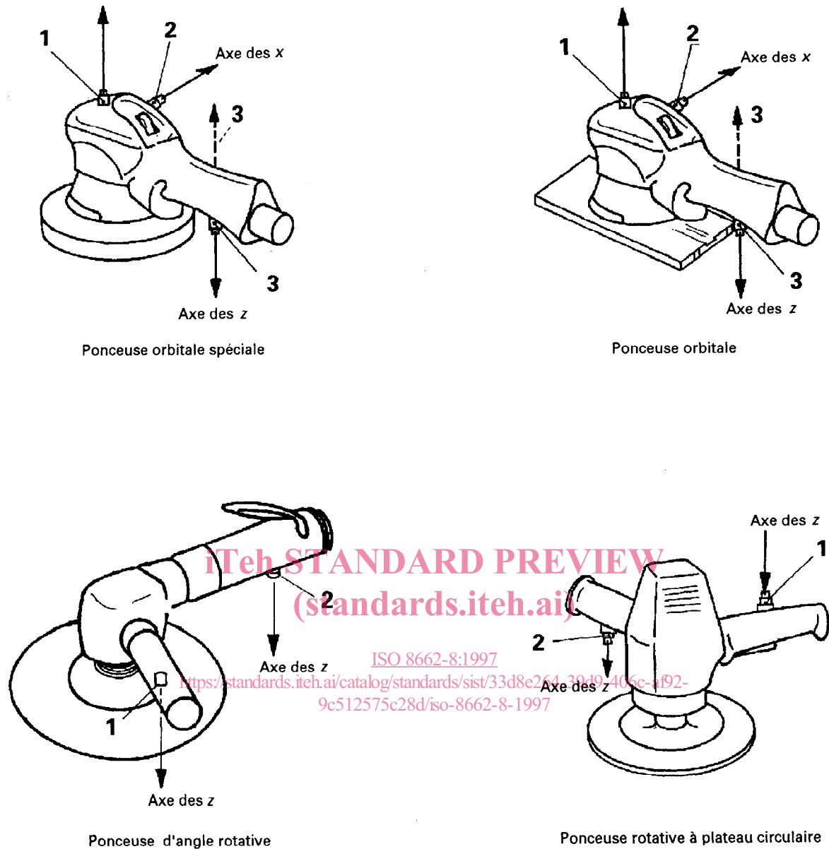
1, 2, 3: Position des transducteurs
