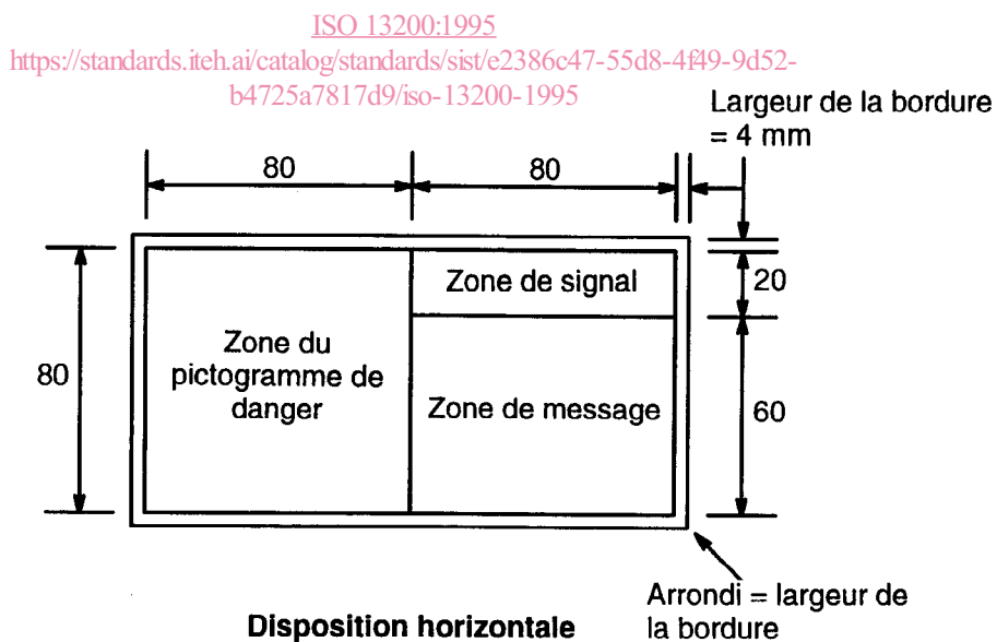
Figure 11 — Dimensions recommandées pour le format à trois zones comportant une zone de signal, une zone de pictogramme et une zone de message
