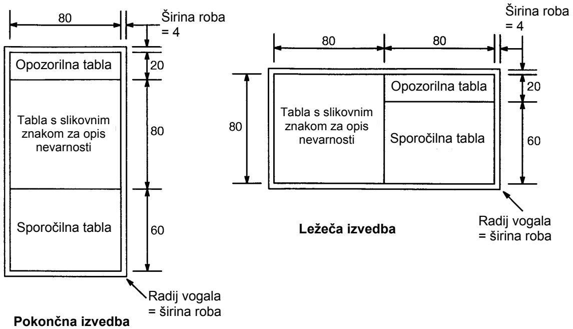
Slika 11: Priporočene mere: tridelna oblika: opozorilna tabla, tabla s slikovnim znakom, sporočilna tabla
