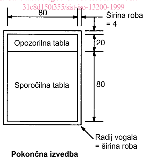
Slika 10: Priporočene mere: dvodelna oblika: signalni del, sporočilni del
