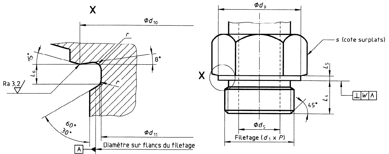
Figure 1 — Élément mâle avec étanchéité métal sur métal (type B)
