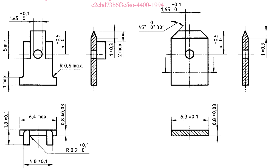
b) Dimensions des broches
