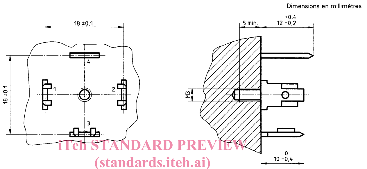
a) Position et marquage des broches et du contact de sécurité
