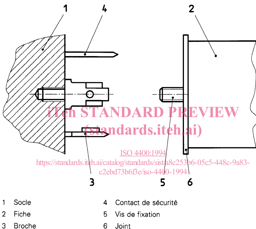
Figure 1 — Composants du connecteur
