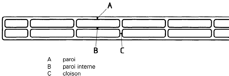
Figure 3 — Exemple de plaque triple paroi
