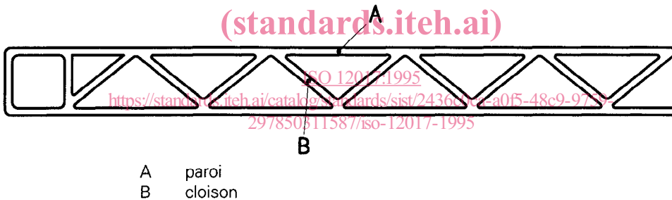
Figure 2 — Exemple de plaque double paroi
