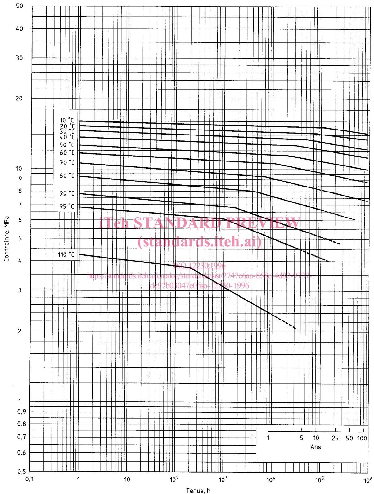
Figure 1 — Résistance espérée des tubes en polybutène (PB)
