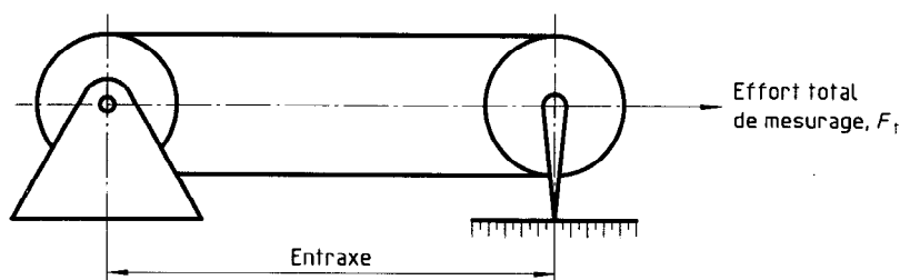
Figure 5 — Appareil de mesurage de la longueur primitive
