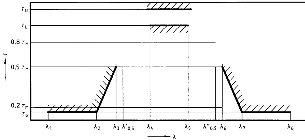
Figure 5 — Fonction filtrante
