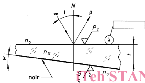
Figure A.1 — Réflectance, faisceau collimaté
