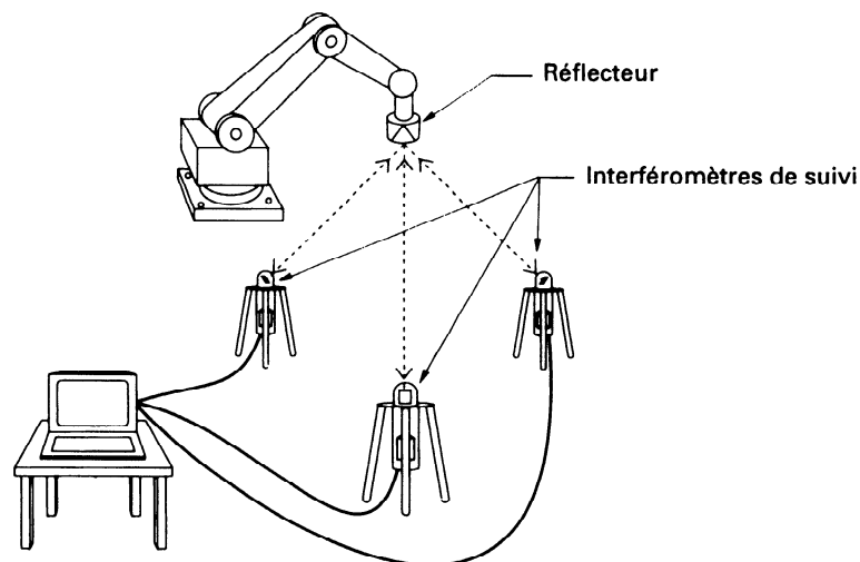
Figure 6 : suivi interférométrique multi-faisceaux
