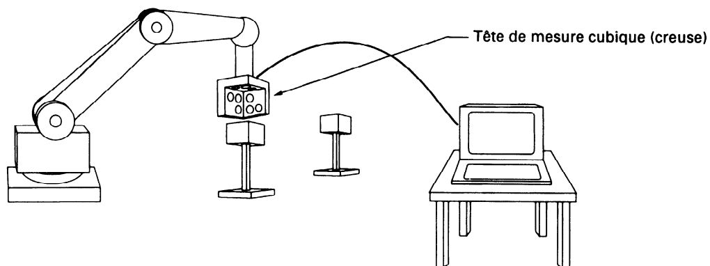
Figure 1 : méthode de positionnement d'une tête de mesure "artefact" (cubique)
