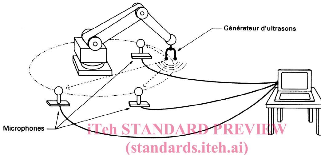
Figure 7 : triangulation par ultrasons
