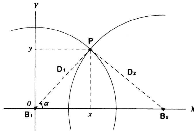
Figure 5 : principe de mesure par triangulation (représentation bi-dimensionnelle)
