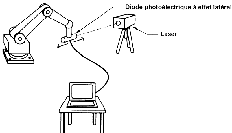
Figure 4 : comparaison de trajectoire par faisceau laser
