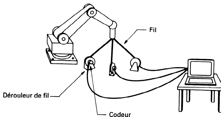
Figure 8 : triangulation mécanique par fils
