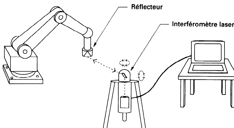
Figure 10 : suivi interférométrique uni-faisceau pour la mesure de la position
