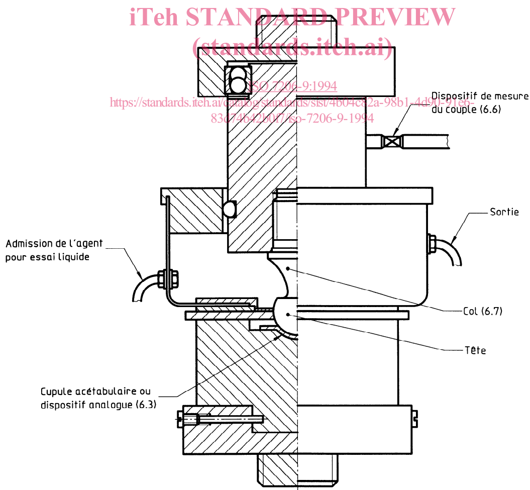
Figure 1 — Exemple d'appareillage utilisé pour déterminer la résistance au couple de l'assemblage tête/col
