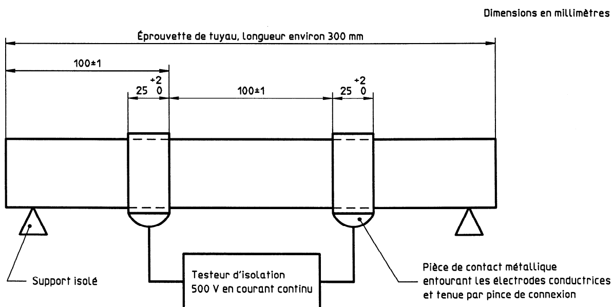
Figure 1 — Électrodes et contacts pour l'essai tels que décrits en 3.5.2.1
