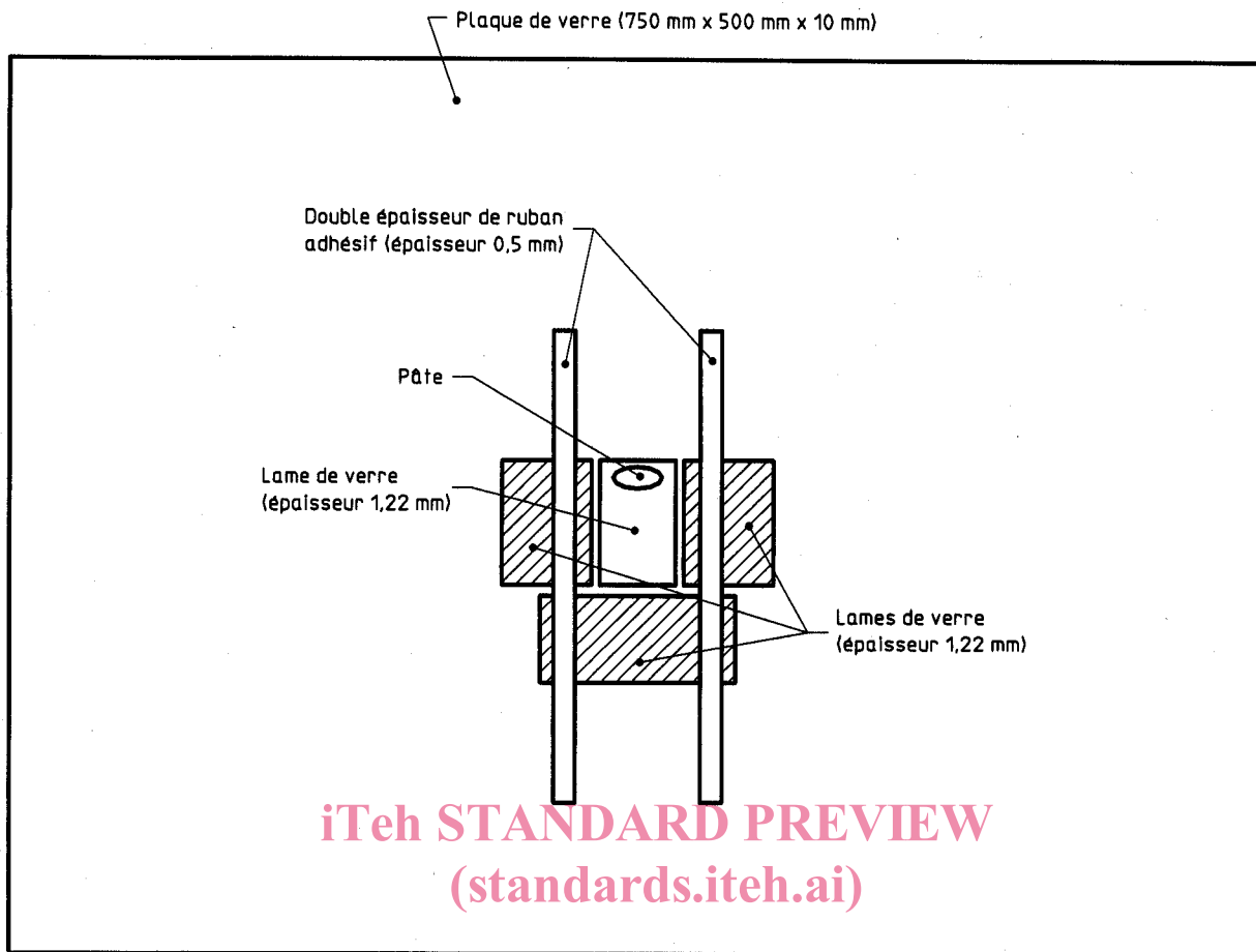
Figure 1 — Dispositif de préparation des lames échantillons pour le Meeco Colormaster
