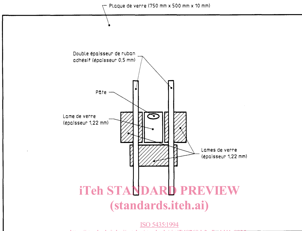
Figure 1 — Dispositif de préparation des lames échantillons pour le Meeco Colormaster
