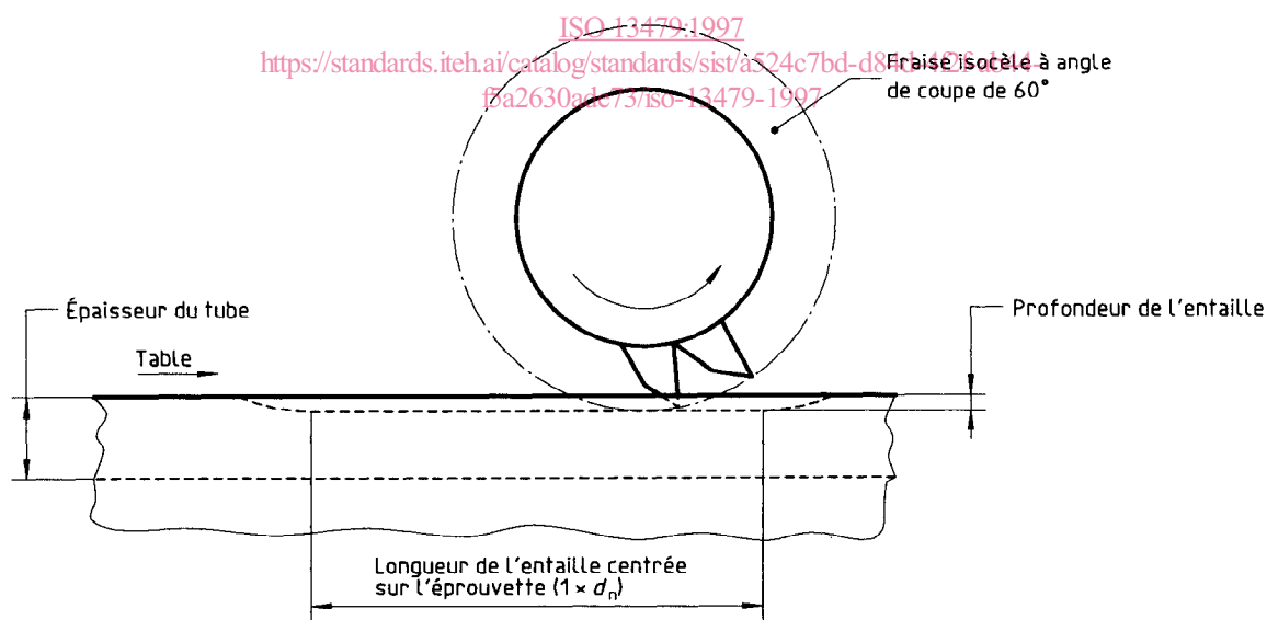
Figure 2 — Méthode d'entaillage
