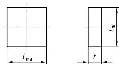
b) Forme WR (fenêtre rectangulaire plane)
