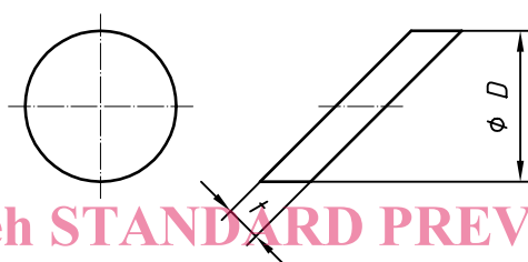
c) Forme WE (fenêtre elliptique plane)
