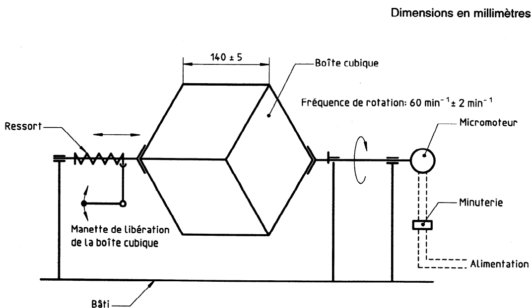
Figure 1 — Boîte rotative cubique (sismélatophore)
