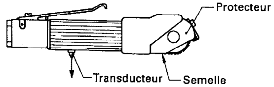
Petite scie circulaire
