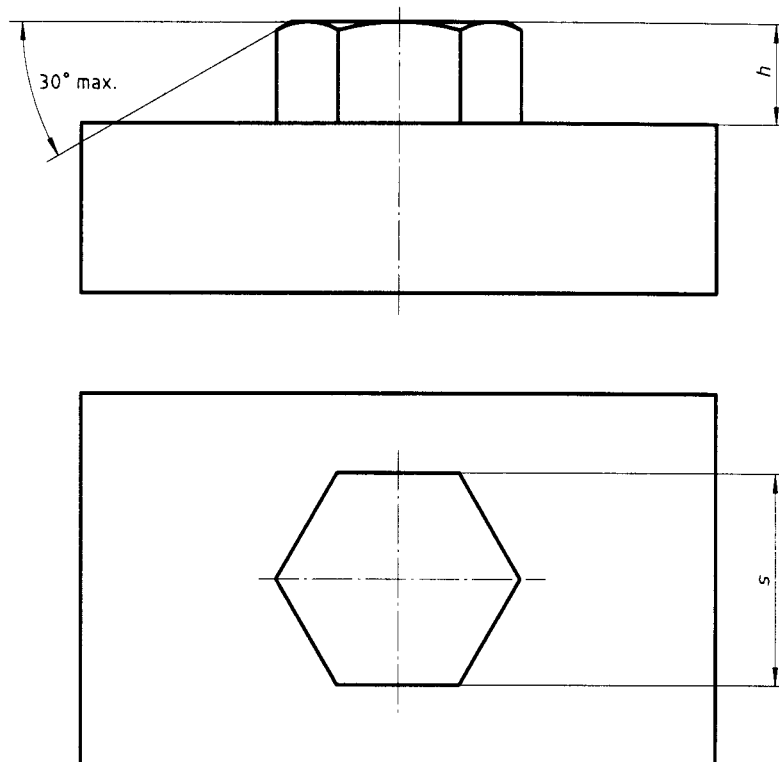
Figure 1 — Hauteur et cote surplats du mandrin d'essai
