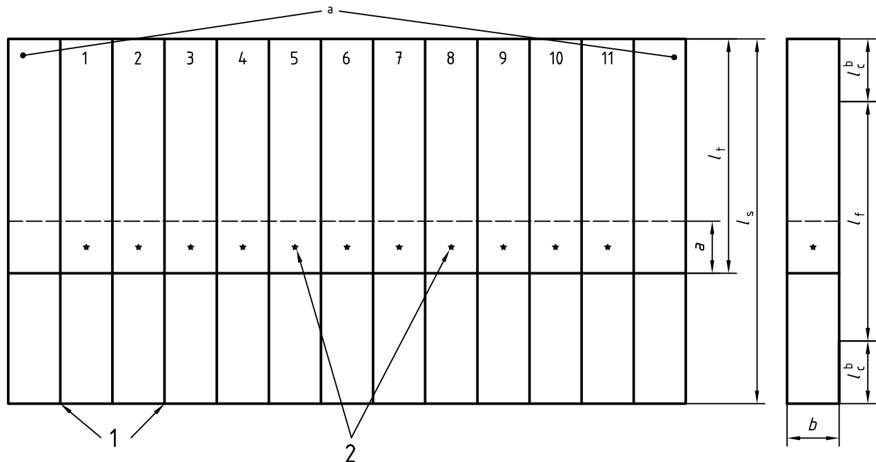
a) Pièce d'essai multipoint
