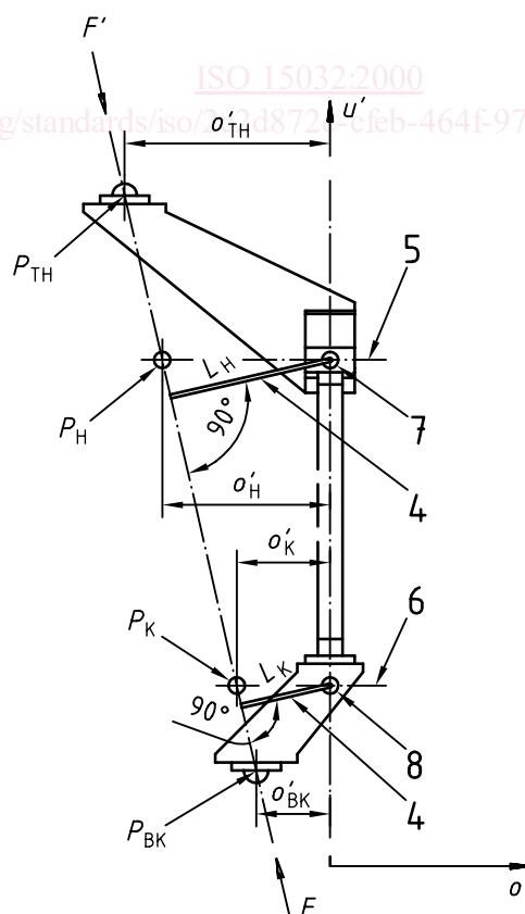
Figure 2 — Configurations d'essai pour les essais A-P et M-L dans les plans f'-u' et o'-u'
