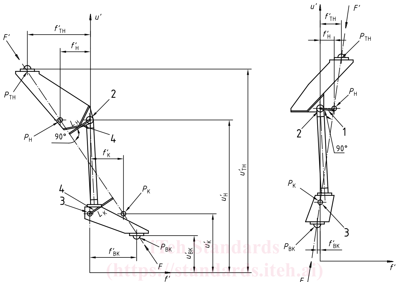
a) Condition de mise en charge d'essai A-P en extension
