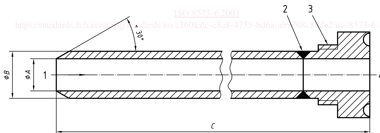
Figure 1 — Montage du matériel d'insertion de la sonde pour le prélèvement
