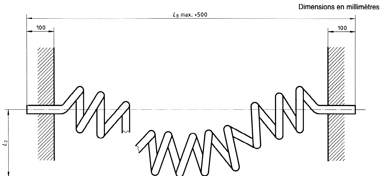
Figure 1 — Mesurage de la flèche du câble
