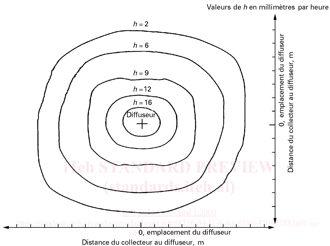
Figure 6 — Isoplèthes des hauteurs d'eau appliquées sur la surface arrosée
