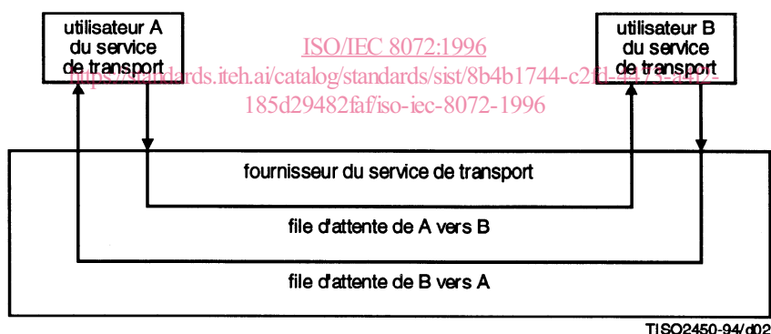
Figure 1 – Modèle abstrait d'une connexion de transport
