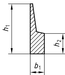
Figure 1 — Profil de type A
