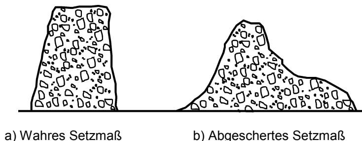
Bild 2 — Formen des Setzmaßes
