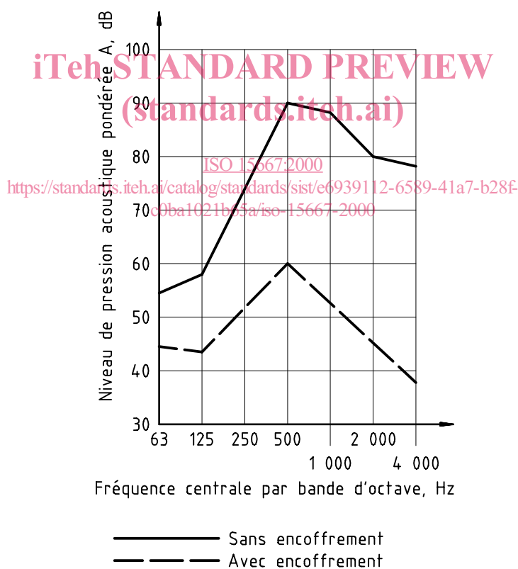
Figure 3 — Exemple type d'un spectre par bandes d'octave pondéré A du niveau de pression acoustique au voisinage d'une machine
