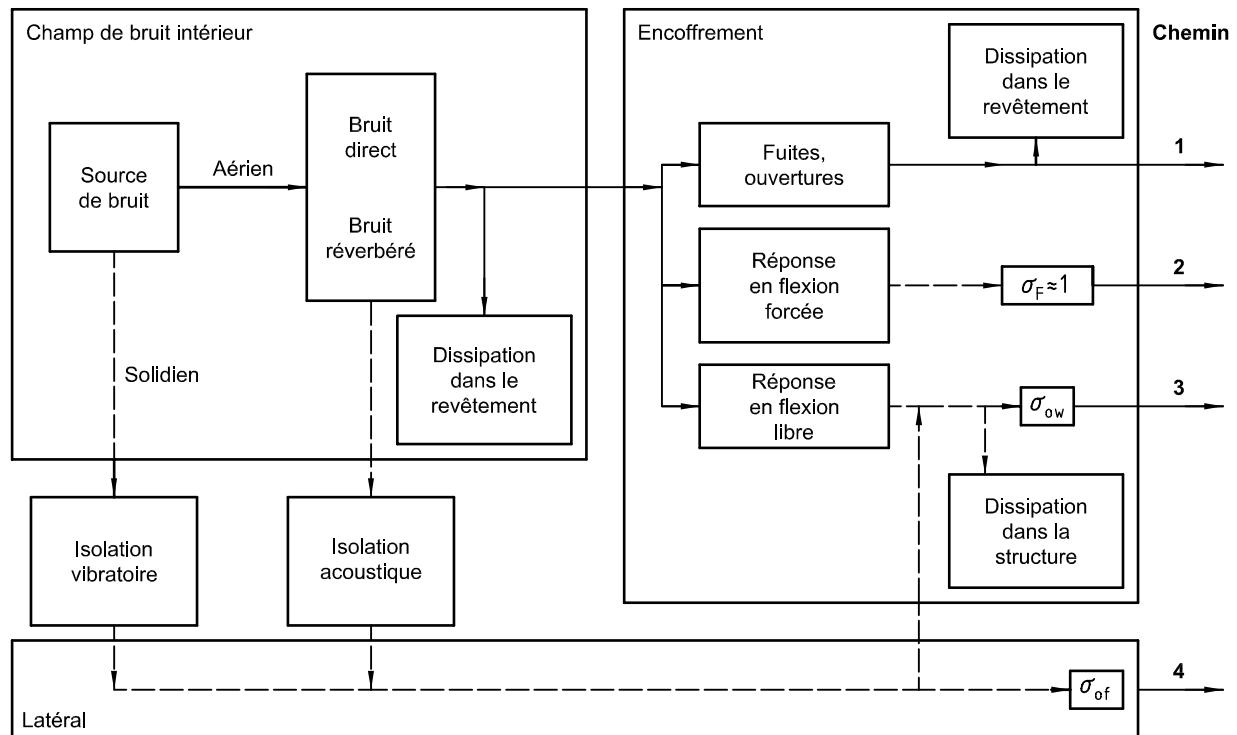
Figure 1 — Schéma synoptique des chemins de propagation du son
