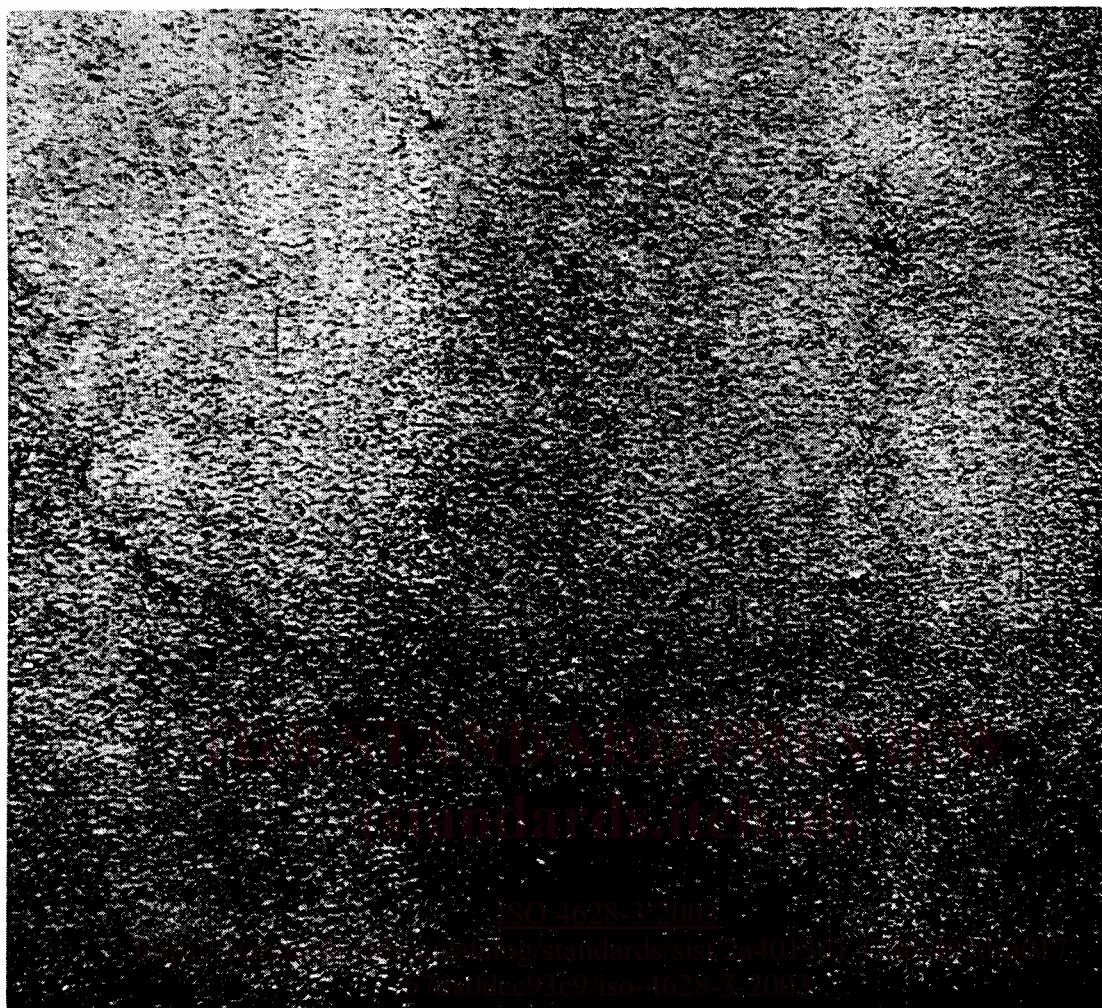
Рисунок 1 — Степень ржавления Ri 1
