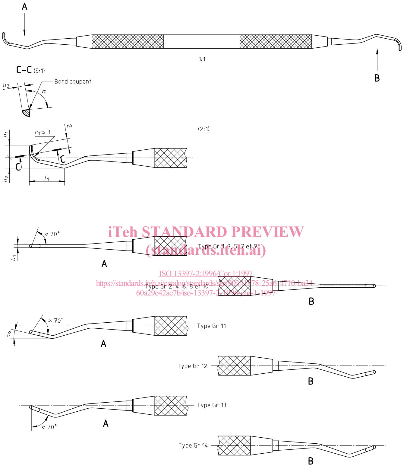
Figure 1 — Curettes parodontales — Types Gr 1 à 14
