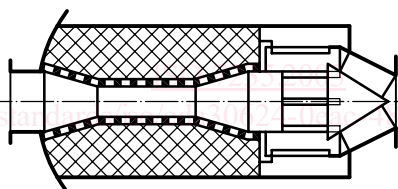
e) Silencieux à pare-étincelles
