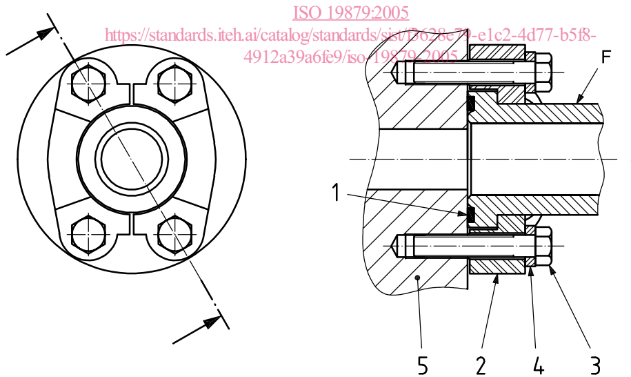
Figure 3 — Autre montage d'essai de capacité du connecteur en l'absence de tube — Type 3
