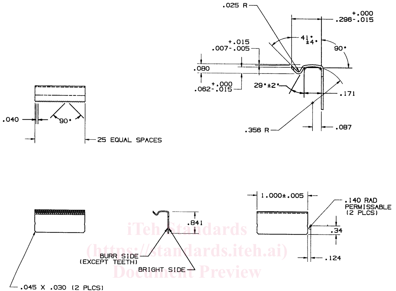
FIG. 1 Blade
