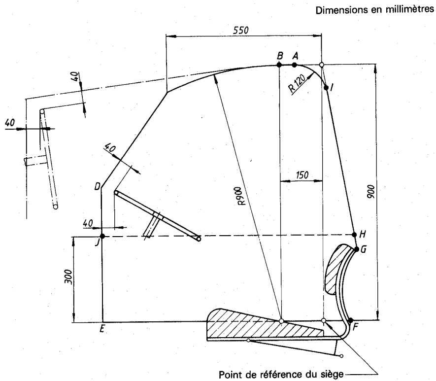
Figure 2a) — Zone de dégagement vue de côté
