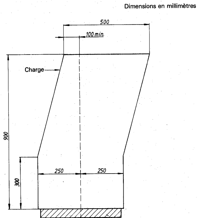
Figure 2b) — Zone de dégagement vue arrière/avant à 150 mm en avant du point de référence du siège
