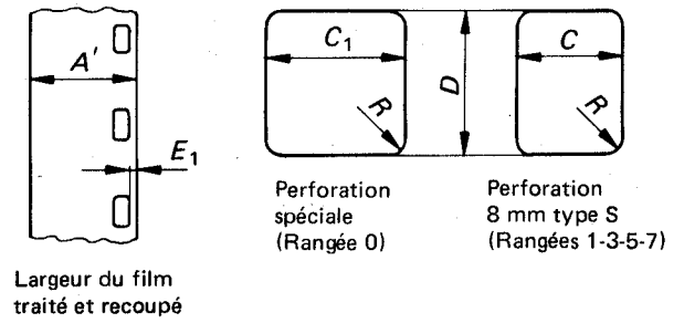
FIGURE 3 – Largeur du film traité et recoupé, et détail des perforations
