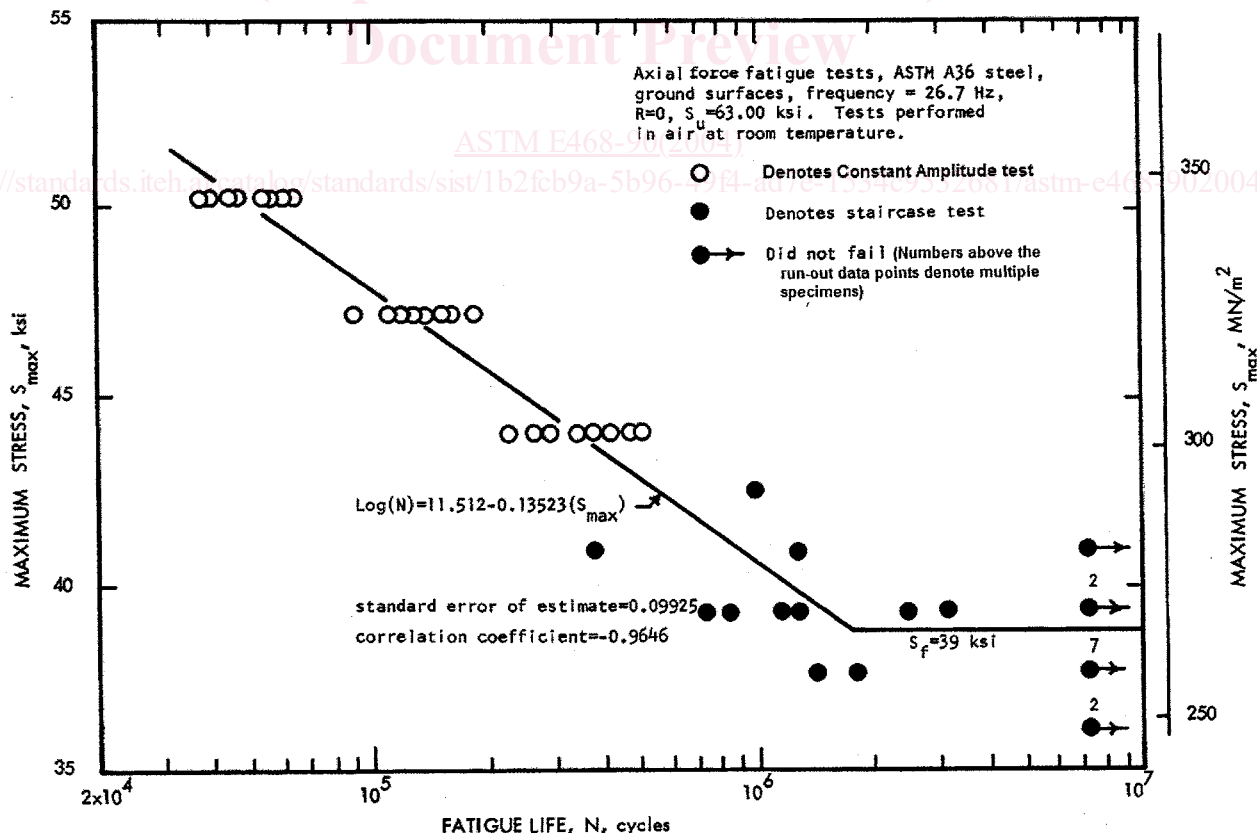
FIG. 1 S-N Diagram
